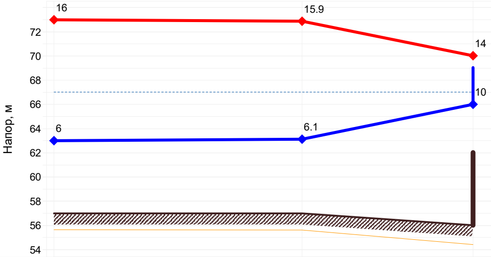
Пьезометрический график от «Кот.№56а» до «МБОУ СОШ №25»
