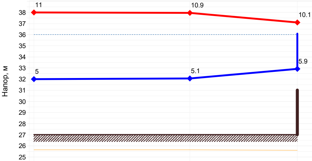
Пьезометрический график от «Кот.№72а» до «МБОУ СОШ №16»
